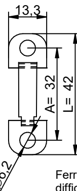
Ferrure droite
