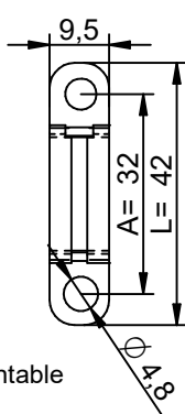
Ferrure droite
