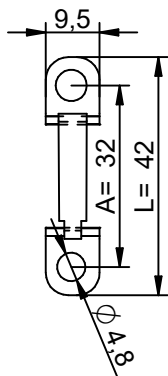
Ferrure gauche facilement démontable
